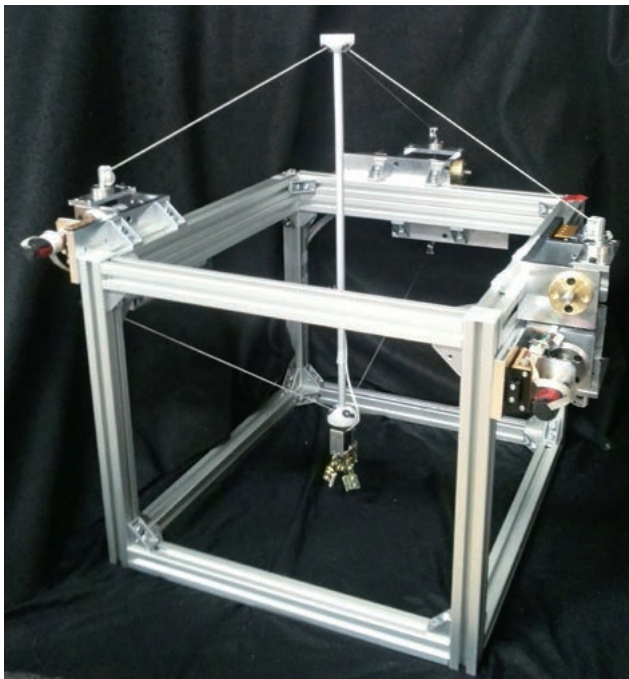
① 6本ワイヤを用いた5DOFのパラレルワイヤ駆動ロボット
